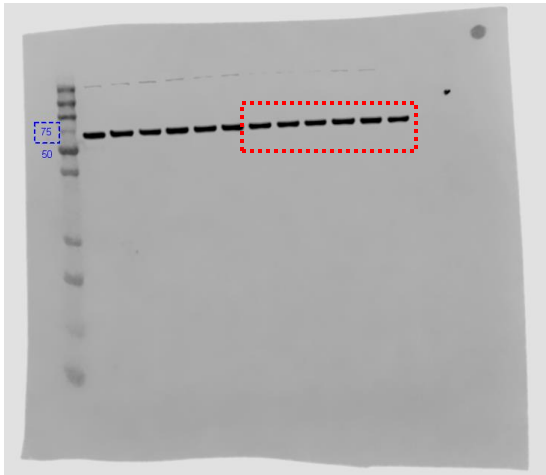
Figure 6E PGC1a
