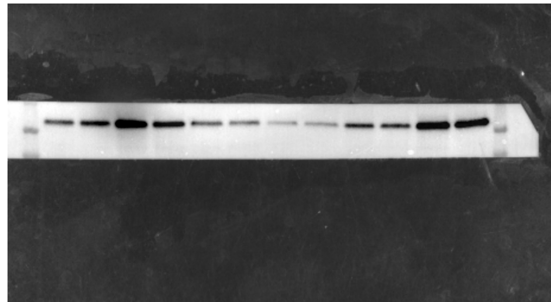
p62 (62 kDa)
