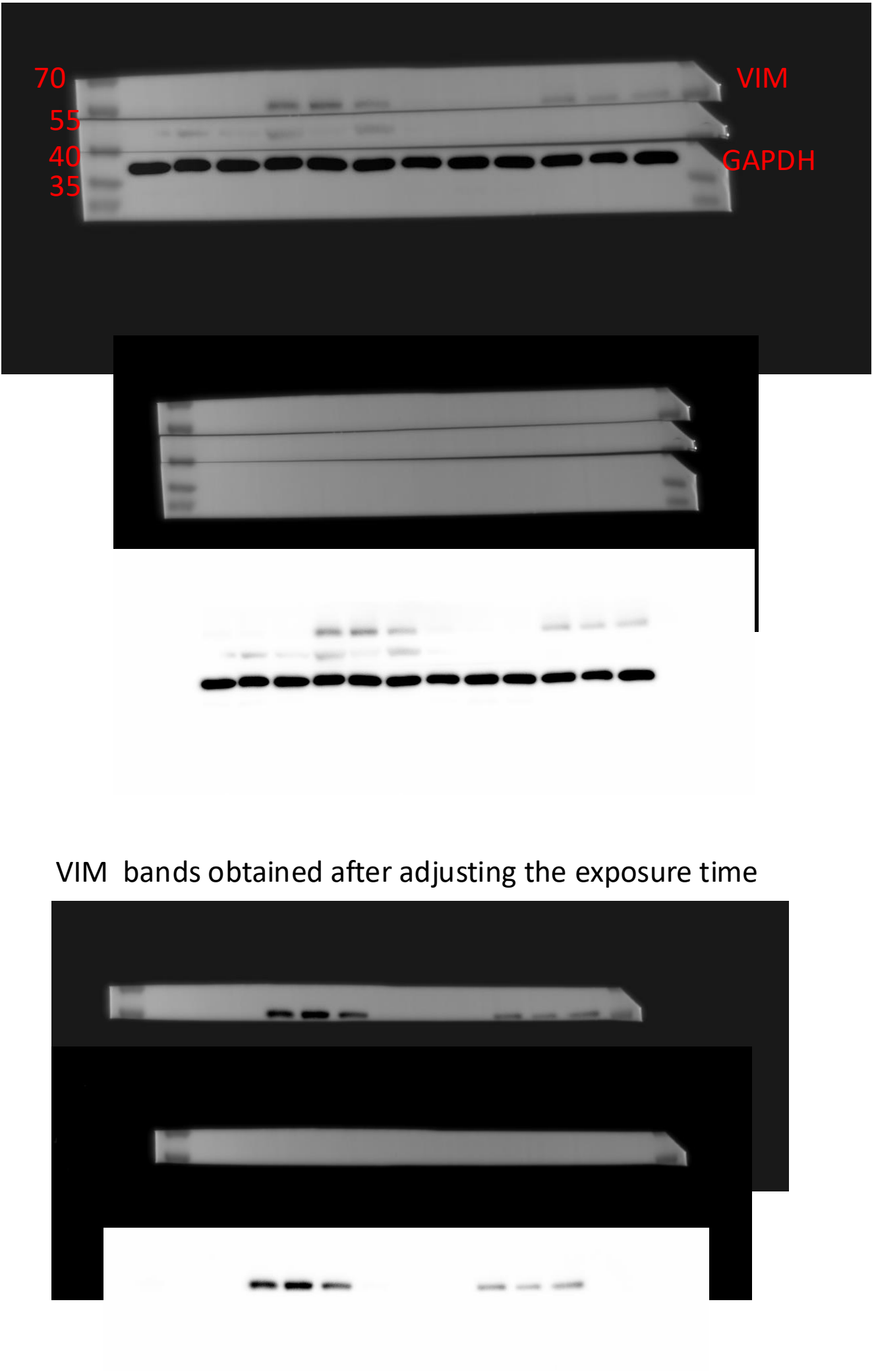
Figure 7E VIM
